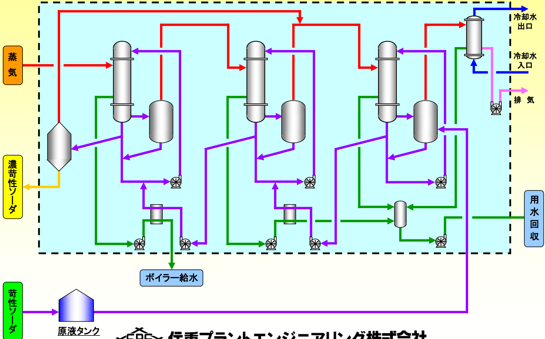
エバポレーター (3重効用)
